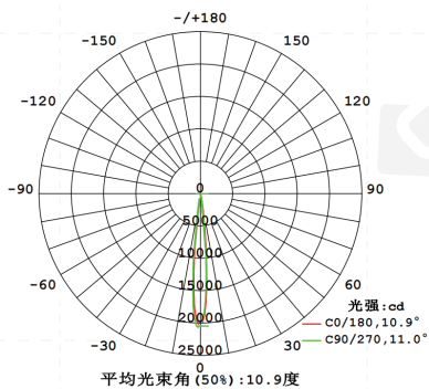
配光曲线图
