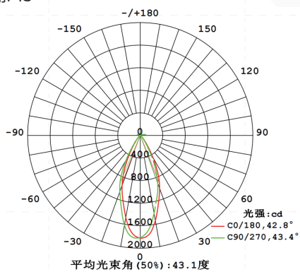
配光曲线图
