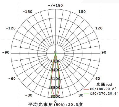
配光曲线图
