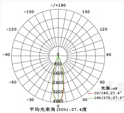
配光曲线图
